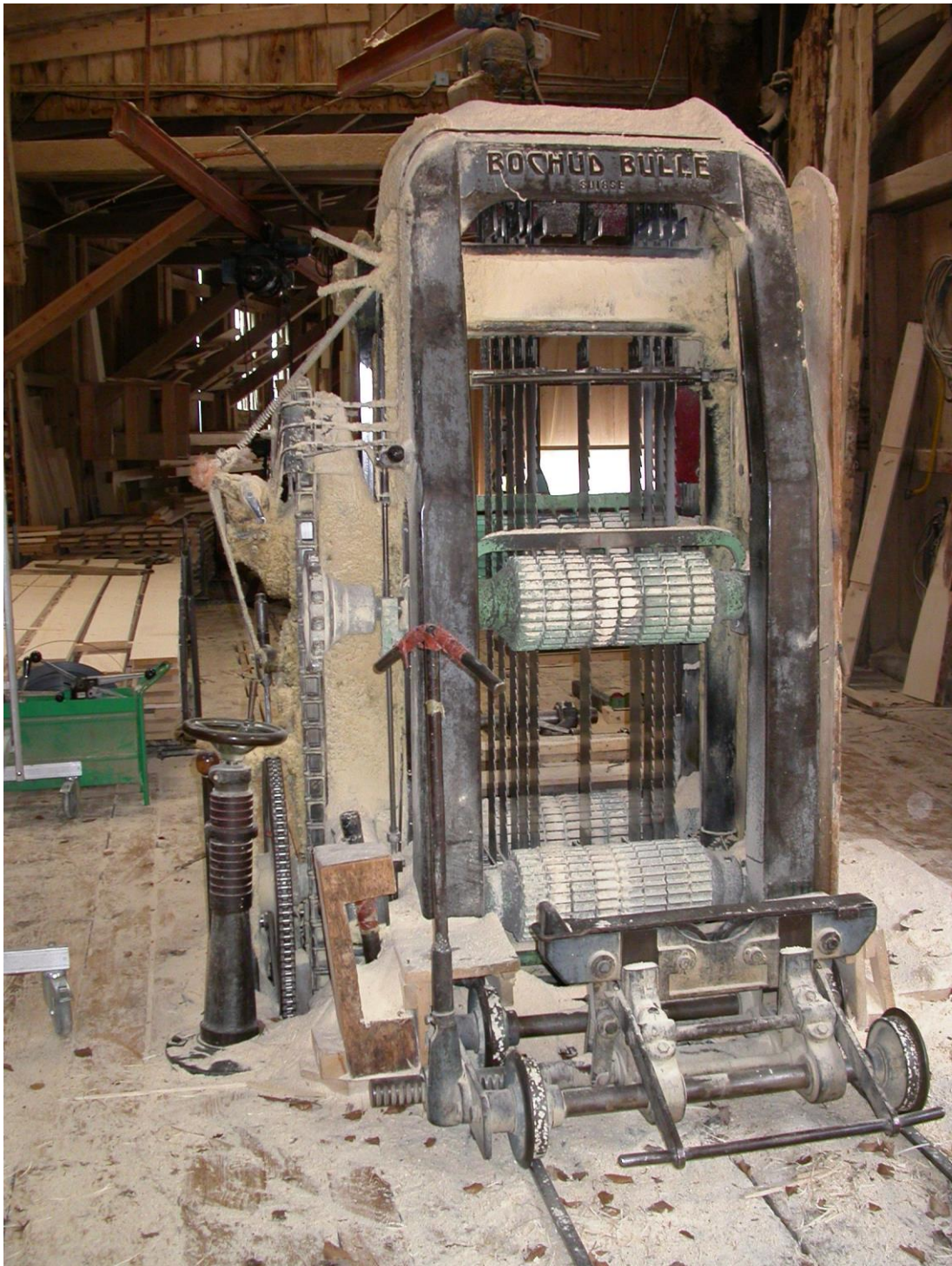
La multiple, merveille de mécanique. Au devant, l'un des deux chariots.
