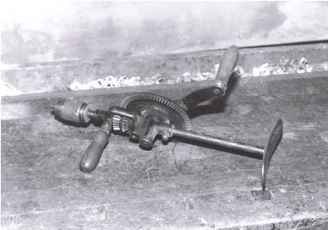
Chignole.
