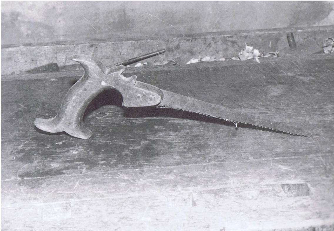
Queue de rat.
