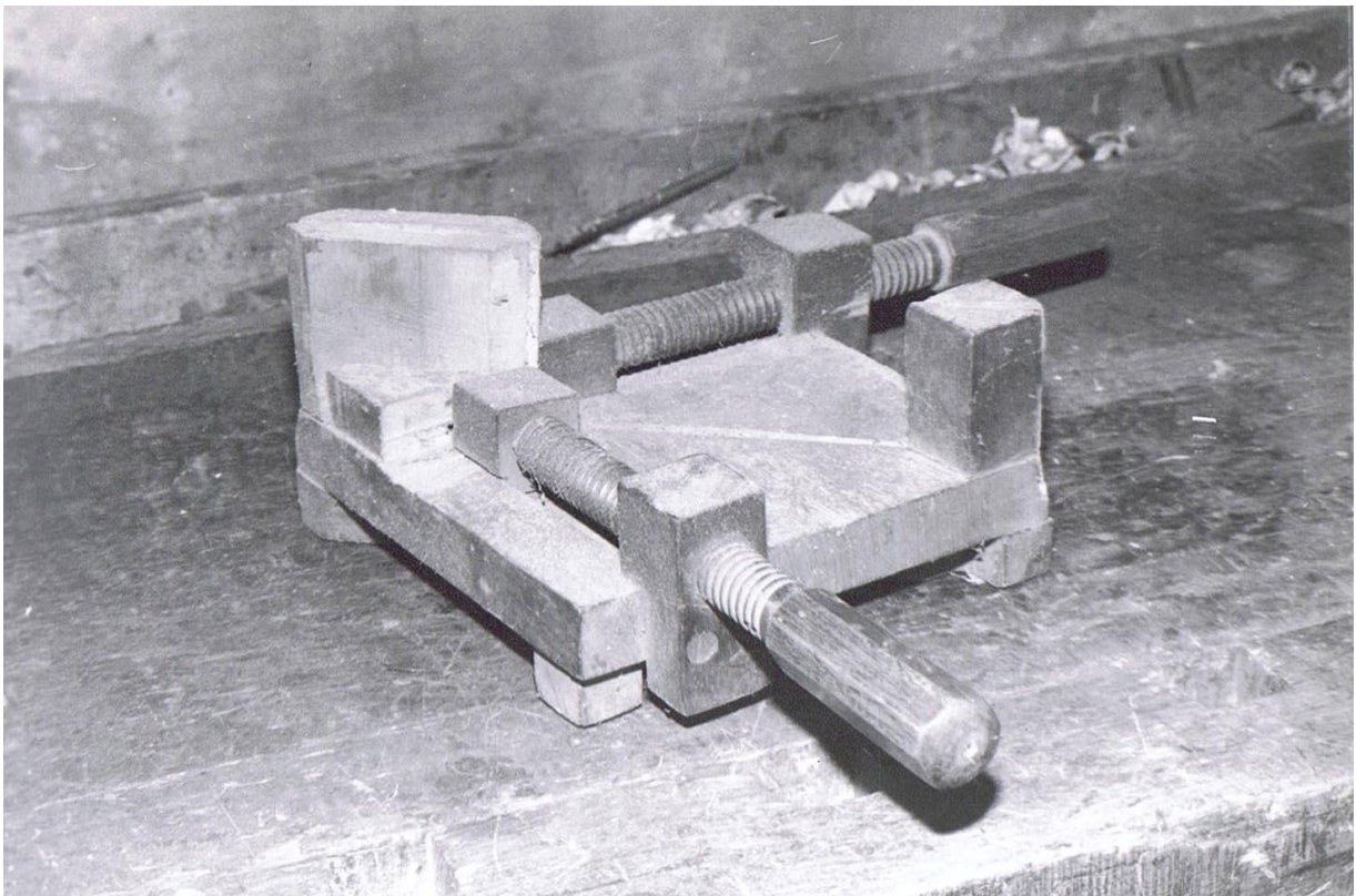
Serre-joint d'une espèce toute particulière.
