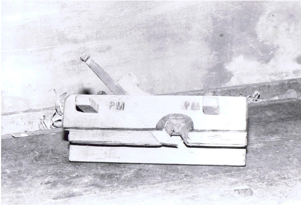
Des rabots en somme de toutes provenances et pour tous usages. Rabet à rainures.
