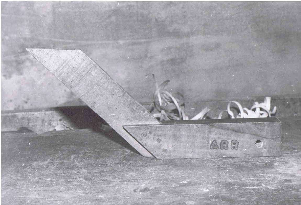
Fausse équerre. ARR = Arthur Rochat, frère de Millet.
