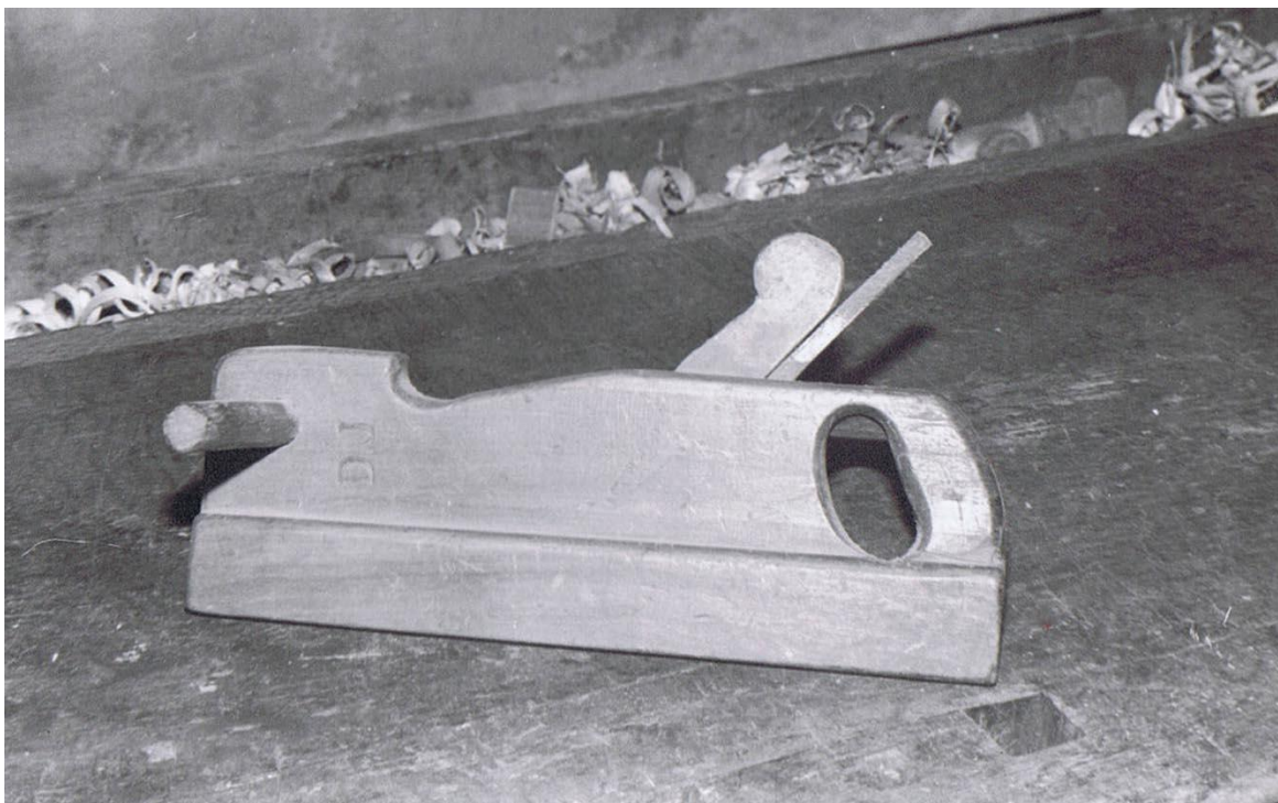
Des rabots en somme de toutes provenances et pour tous usages. Rabet à rainures.
