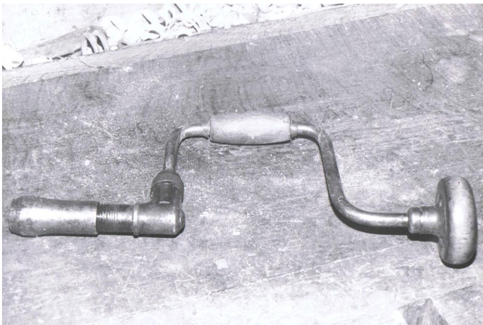
Vilbrequin.
